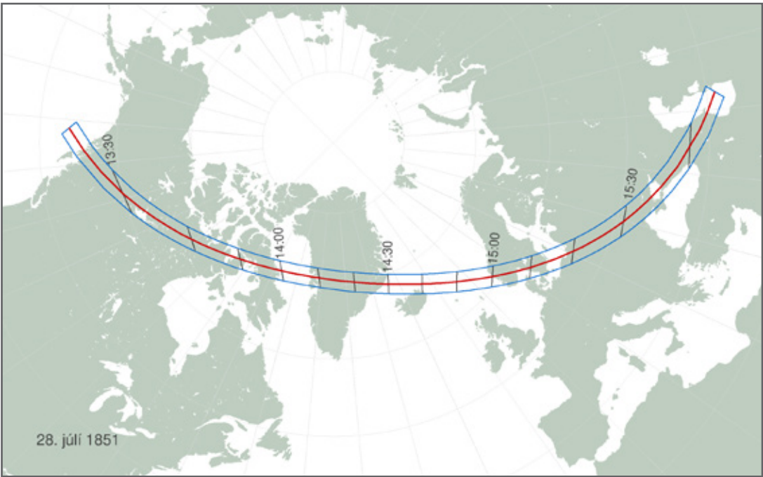
9. mynd. Braut almyrkva á sólu 28. júlí 1851. Almyrkvinn afmarkaðist af bláu línunum og tímasetning er sýnd miðað við íslenska klukku. Almyrkvinn sást við sólarupprás á Kyrrahafi út af Alaska, fór yfir norðausturhluta Íslands um kl. 14.40 og sást síðast við sólsetur á Kaspíahafi. – Path of the total eclipse of the Sun on 28 July 1851. Totality was seen between the blue lines, UTC-times shown. The eclipse started at sunrise over the Pacific off Alaska, went over NE-Iceland at about 14:40 and was last seen at sunset in the Caspian Sea. Kort/Map: Þórður Arason.
