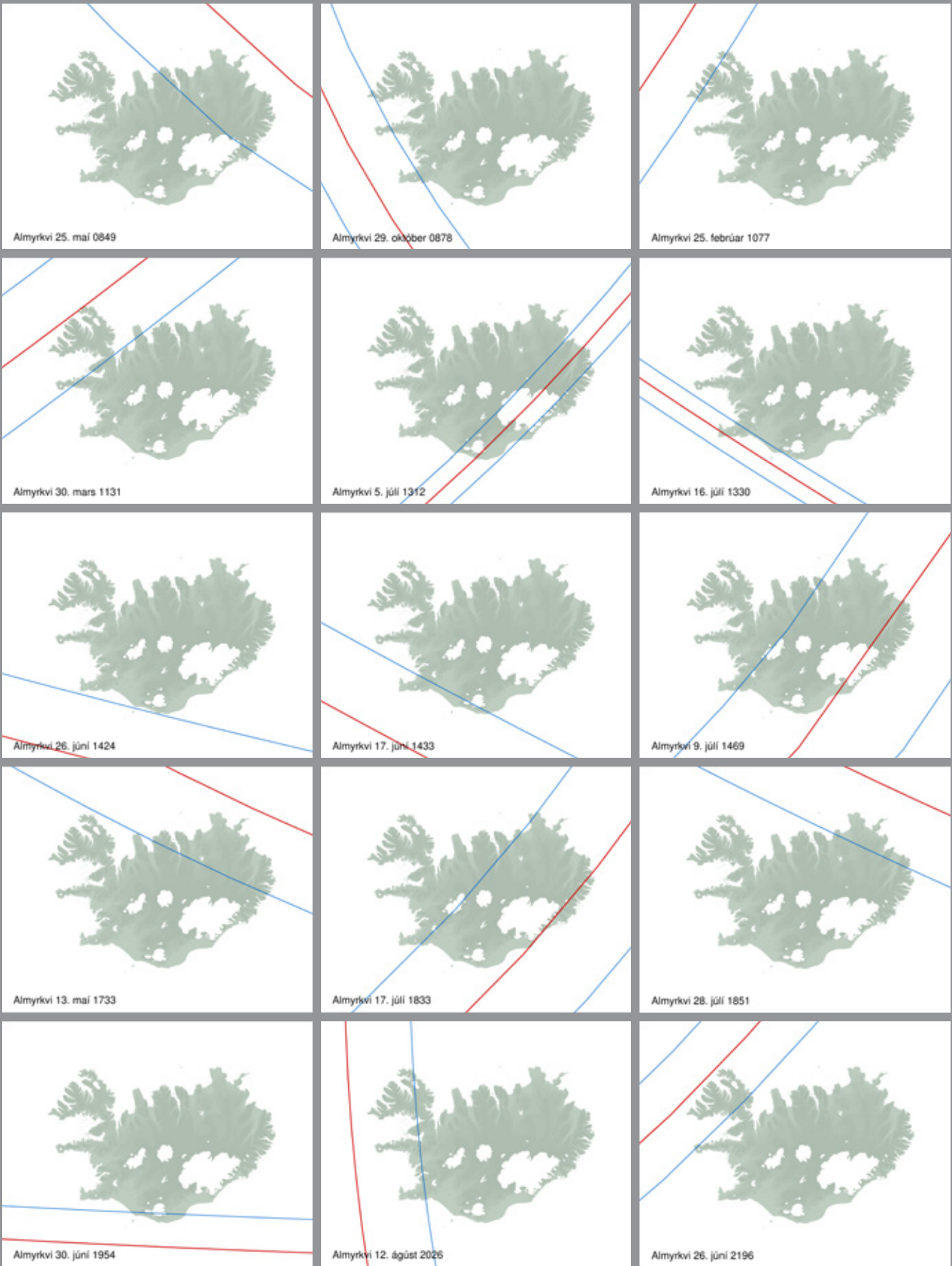
3. mynd. Brautir allra almyrkva á sólu sem fóru/fara yfir Ísland frá 600 til 2200 e.Kr. Hver almyrkvi afmarkast af bláu línunum og miðja myrkvans er á rauðu línunni. – Path of all total eclipses of the sun over Iceland from AD 600 to 2200. Kort/Maps: Póður Arason.
