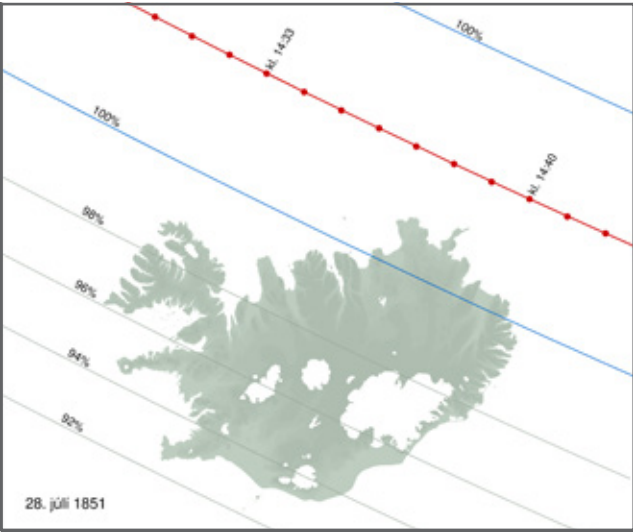
10. mynd. Braut almyrkvans 28. júlí 1851. Almyrkvinn afmarkaðist af bláu línunum og miðja hans var á rauðu línunni. Punktar á rauðu línunni sýna miðju almyrkvans á mínútu fresti. Við hámark varð myrkvun á landinu frá 92% til almyrkvunar á norðausturhluta landsins. – Path of the total eclipse of the Sun on 28 July 1851 over NE-Iceland. The totality occurred between the blue lines. Location of the center of the eclipse is shown at 1 min intervals on the red central line. At maximum the Sun's obscuration was from 92% in SW-Iceland to totality. Kort/Map: Þórður Arason.
