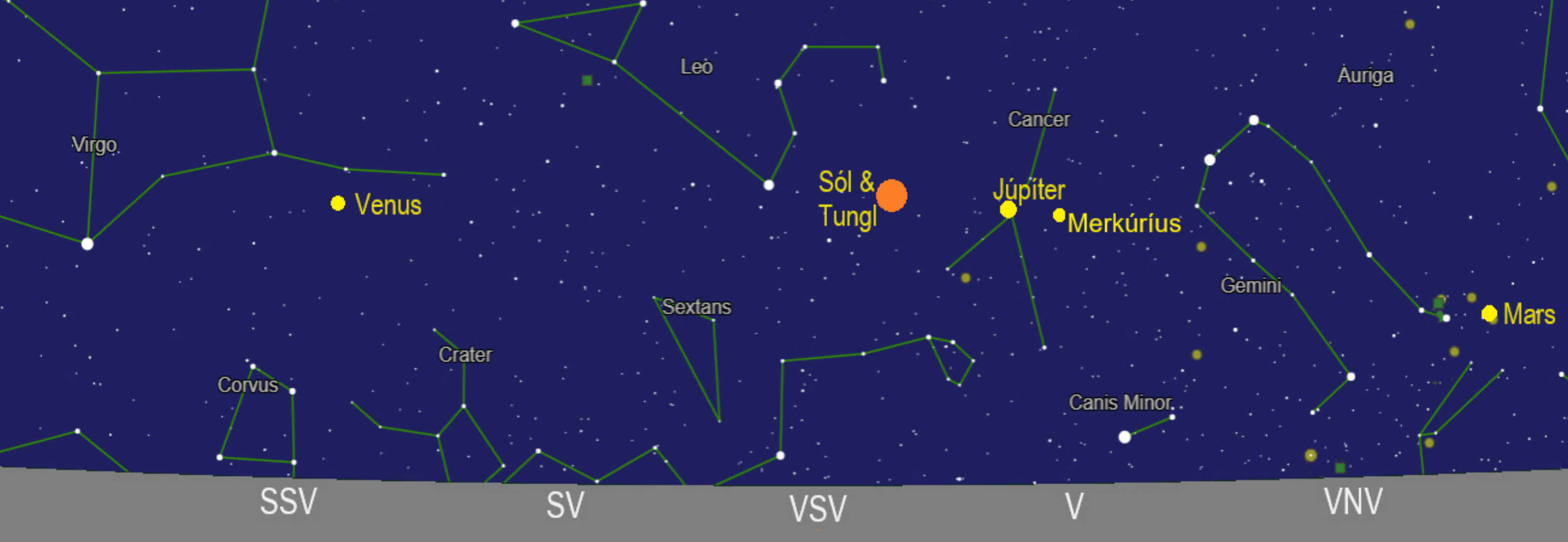
6. mynd. Stjörnukort fyrir Reykjavík í almyrkvanum 12. ágúst 2026, með staðsetningu fjögurra reikistjarna. – Star chart for Reykjavík during the total eclipse on 12 August 2026, with the location of four planets. Mynd/Image: Þórður Arason.
